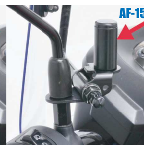
AF-15 ストレートバーΦ22.2 Φ22.2mm x H40mm 汎用クランプなど 取付可能
