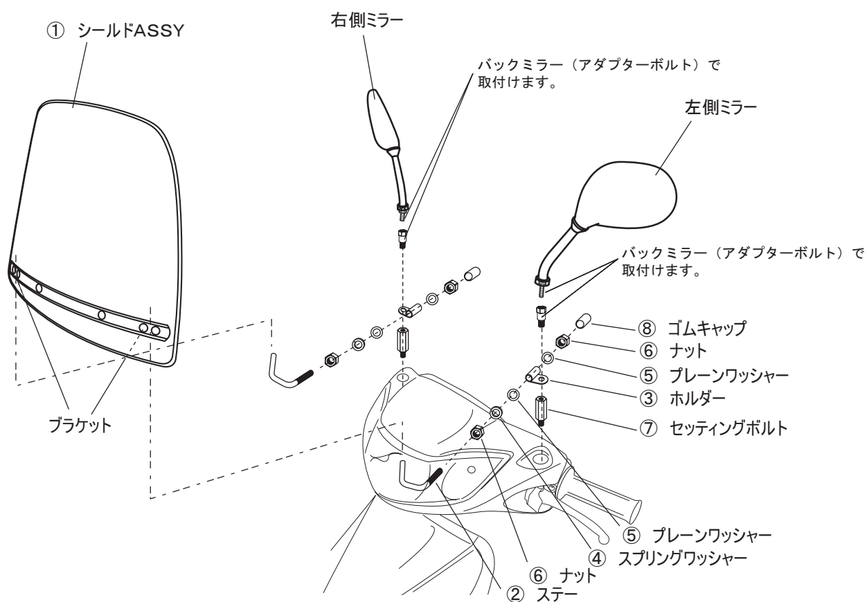
正面図
